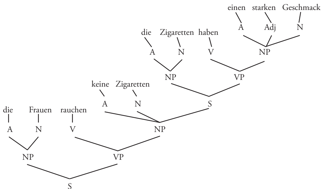
Abbildung 3: Eingebetteter Satz
