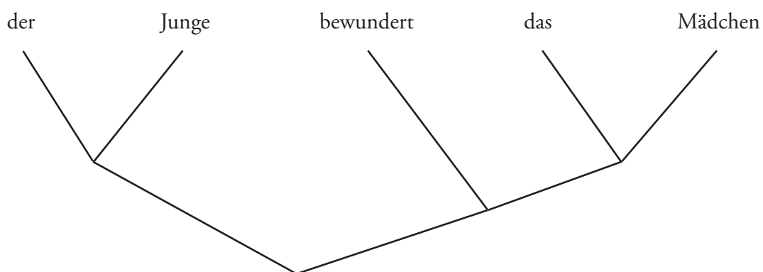
Abbildung 1: Konstituentenstruktur
